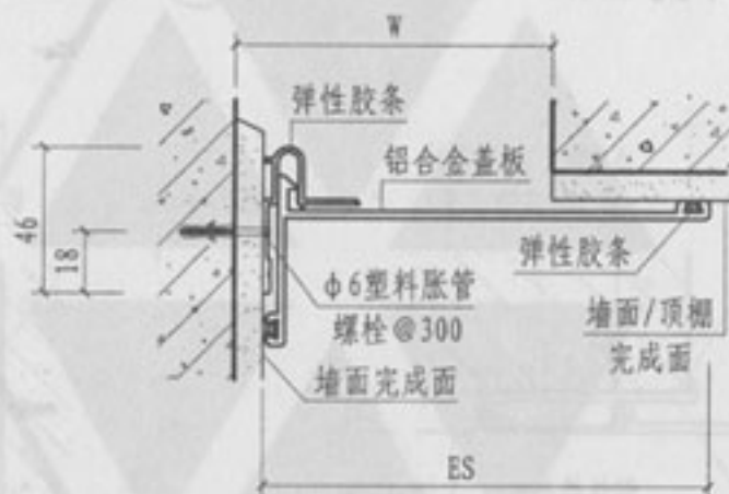
④ 内墙/顶棚 (卡锁式 NJG)
