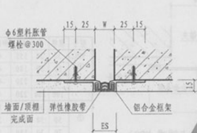
① 内墙/顶棚（嵌平式 NPR）
