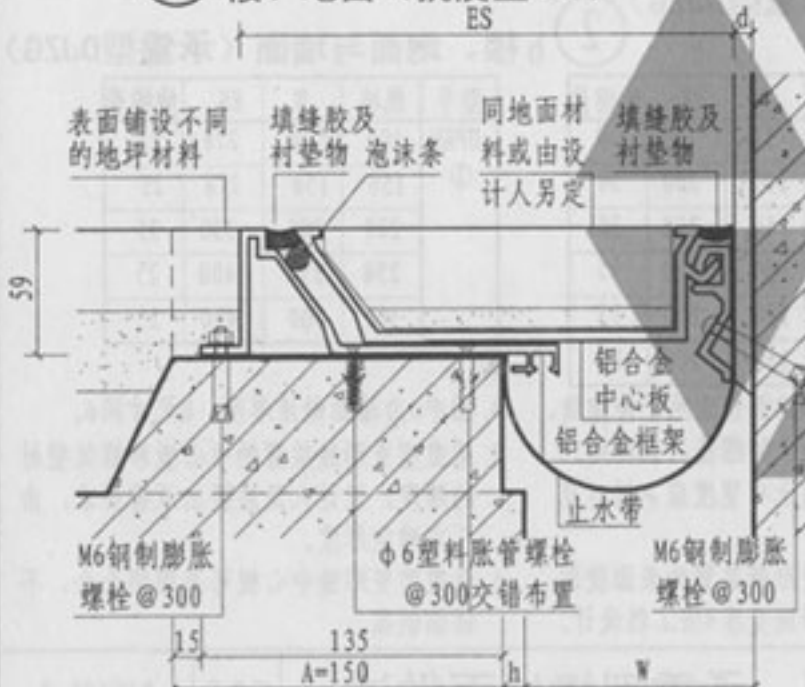
② 楼、地面与墙面 (抗震型DJS)
