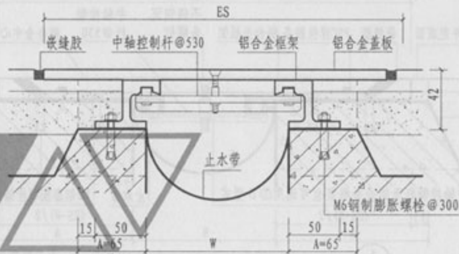
③ 楼、地面（承重型DPZ）
