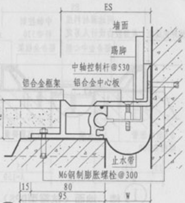
② b 楼、地面与墙面 (承重型DJZG)
