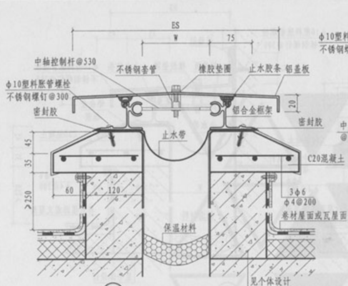
① 屋面 (抗震型 WDP-II)
