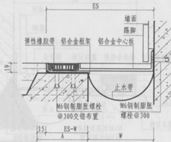
② a 楼、地面与墙面（嵌平式DJRSC）
