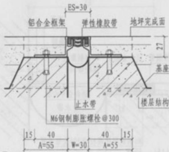
① 楼、地面（嵌平式DPR-30）
