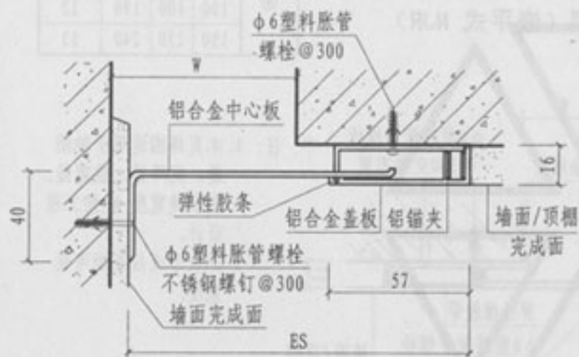
③ 内墙/顶棚 (卡锁式 NJK)
