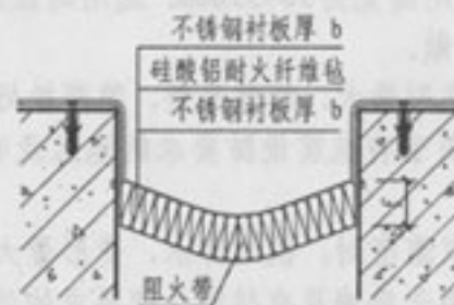
阻火带安装示意图
