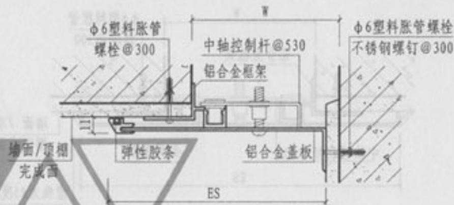
② 内墙/顶棚 (盖板型 NJH)
