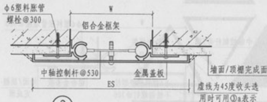
③ 内墙/顶棚 (盖板型 NPL-II)
