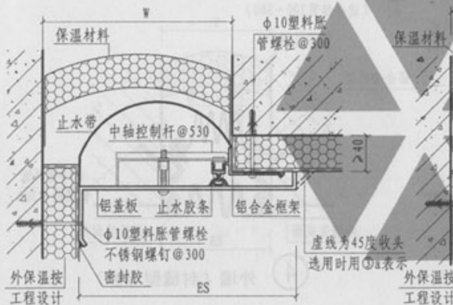
③ 外墙 (盖板型 WQJL)
