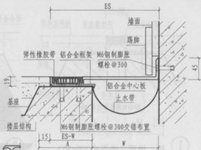
② a 楼、地面与墙面（嵌平式DJR）
