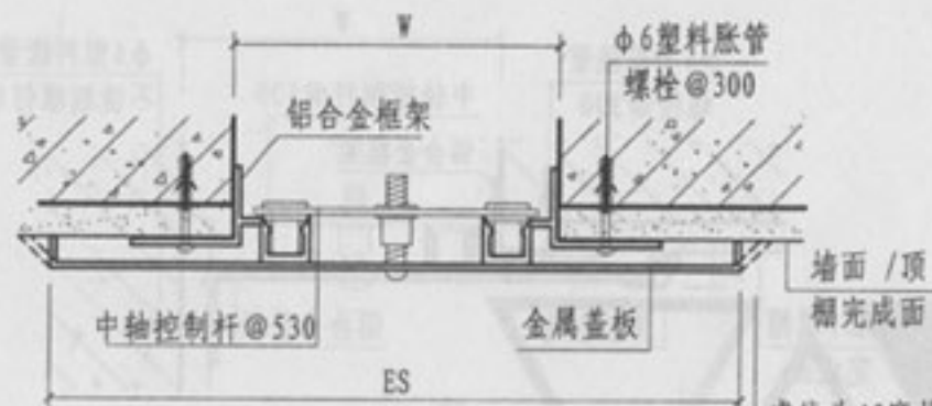
① 内墙/顶棚 (盖板型 NPL)
