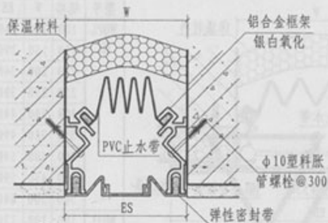
① 外墙（封缝型 WQP） （适合缝宽50-150）
