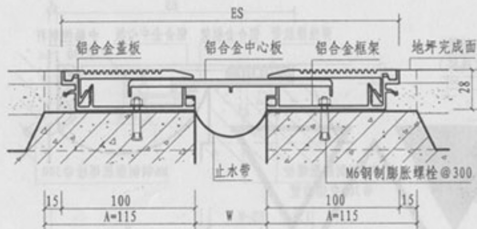
① 楼、地面（卡锁式DPK）
