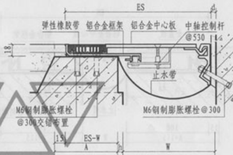
③ 楼、地面与墙面（嵌平式DJC）
