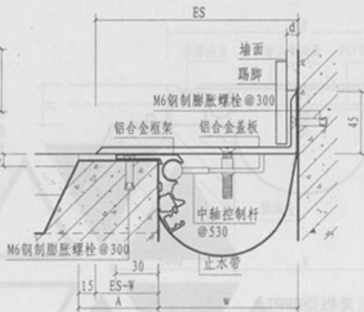
① b 楼、地面与墙面 (盖板型DJLH)
