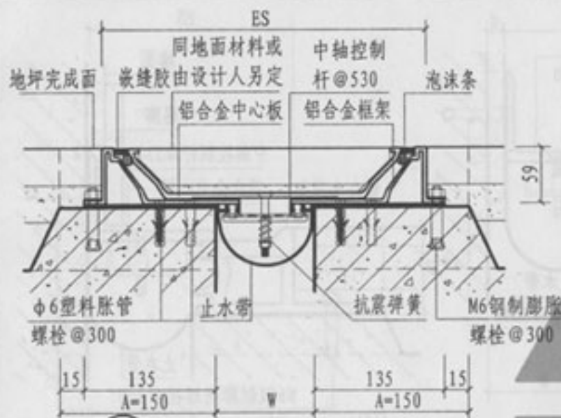
① 楼、地面 (抗震型DPS)
