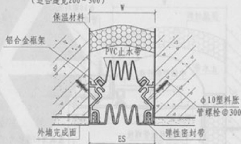
④ 外墙（封缝型 WQR）
