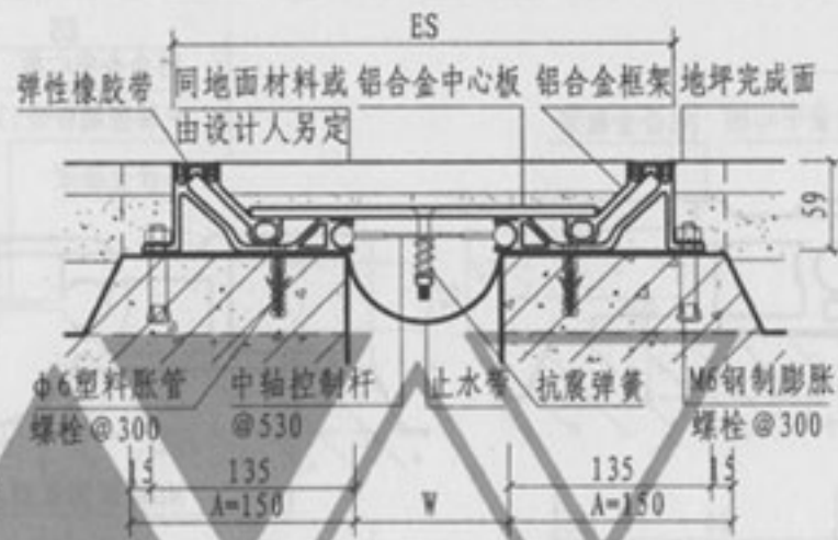
③ 楼、地面 (抗震型DPSM)
