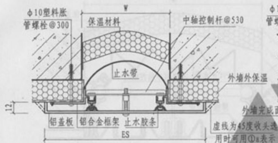
① 外墙 (盖板型 WQPL)
