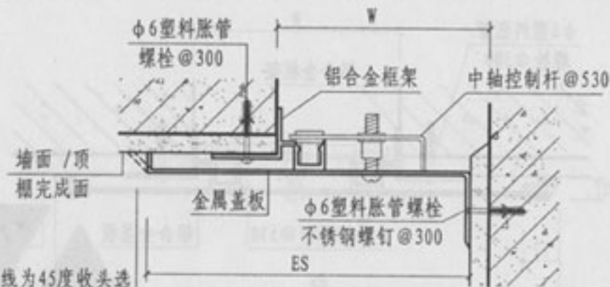
② 内墙/顶棚 (盖板型 NJL)
