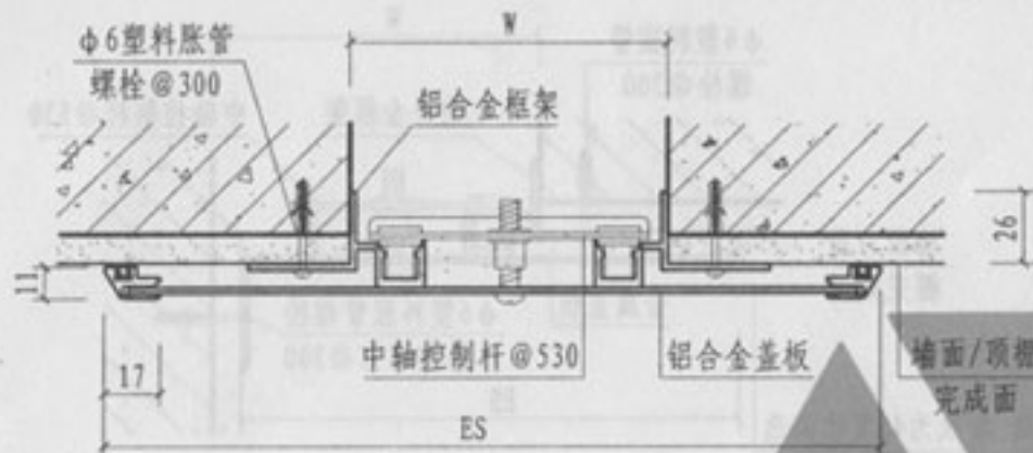
① 内墙/顶棚 (盖板型 NPH)
