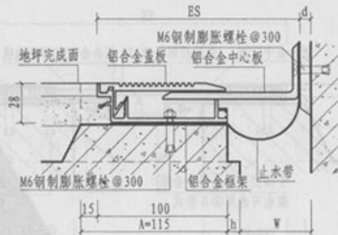
② 楼、地面与墙面（卡锁式DJK）
