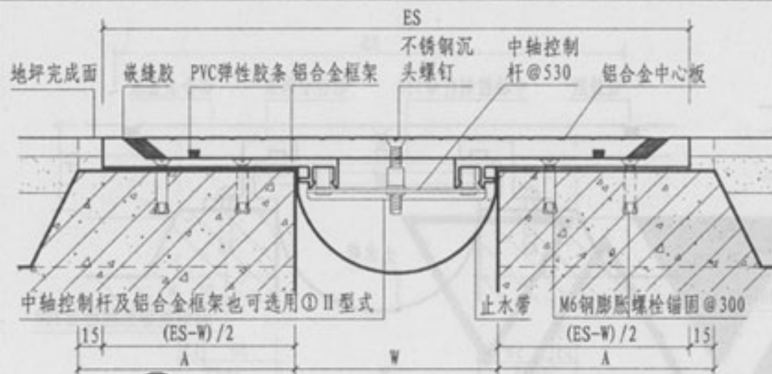
①a 楼、地面（承重型DPZH）
