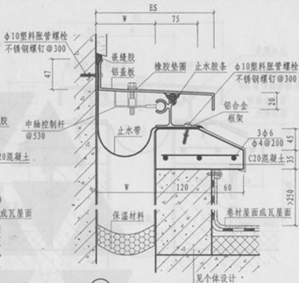
② 屋面 (抗震型 WDJ-II)
