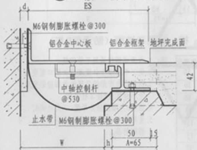
② b 楼、地面与墙面（盖板型DJL）
