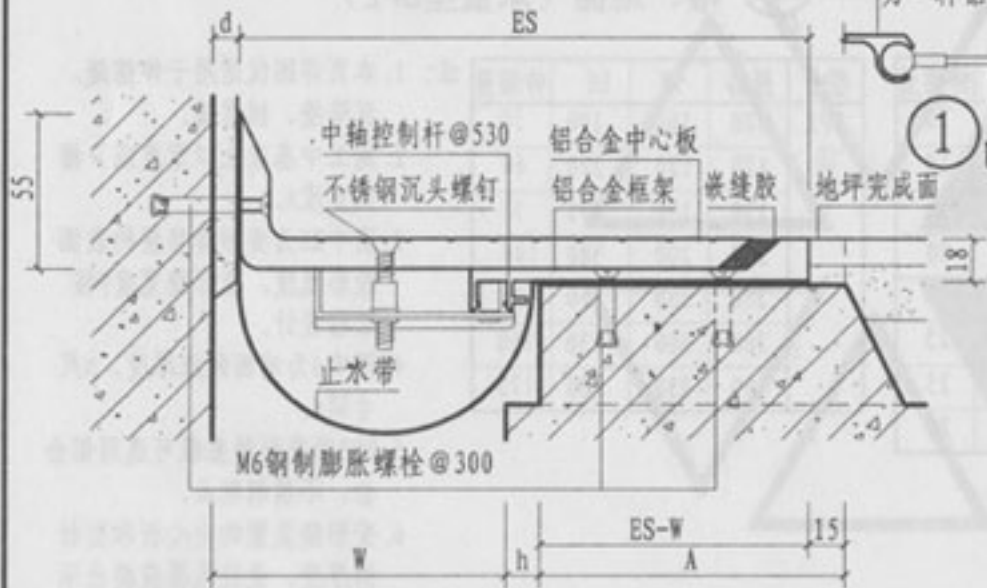
①b 楼、地面（承重型DPZH）
