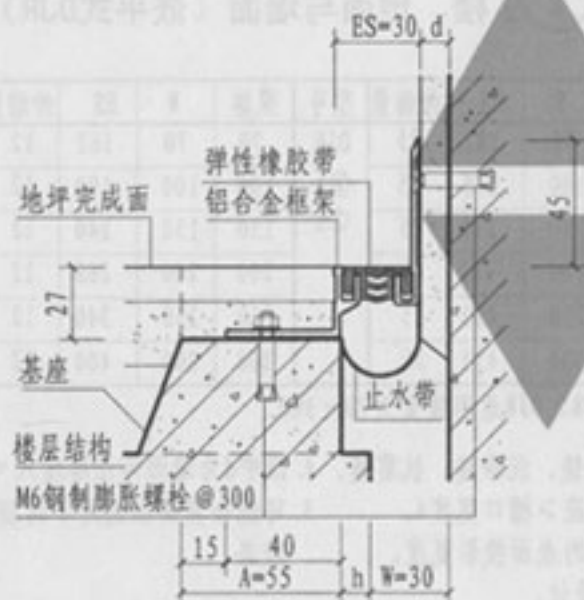
③ 楼、地面与墙面（嵌平式DJR-30）
