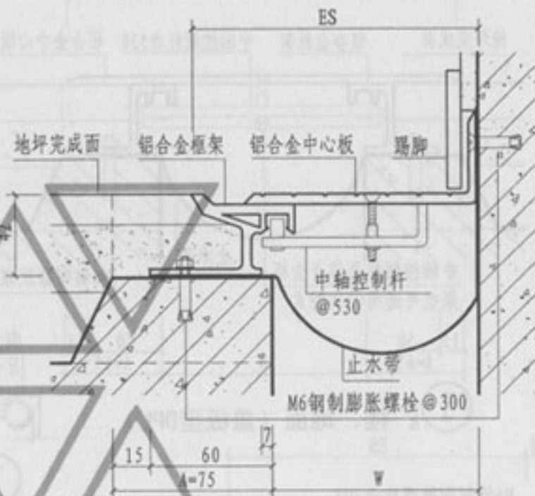
② a 楼、地面与墙面 (防滑型DJF)
