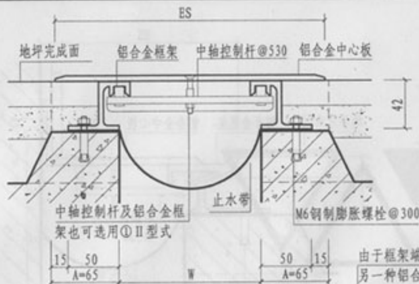
① a 楼、地面（盖板型DPL）
