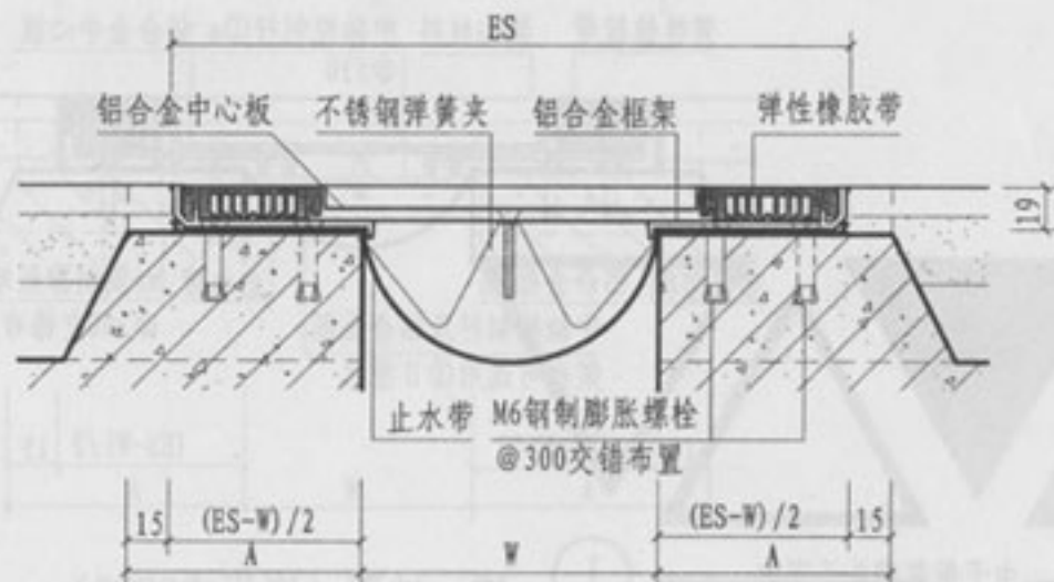
① 楼、地面（双列嵌平式DPRSC）
