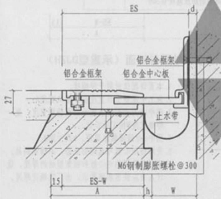
② 楼、地面与墙面（承重型DJZL）
