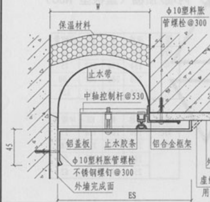
③ 外墙 (盖板型 WQJL)
