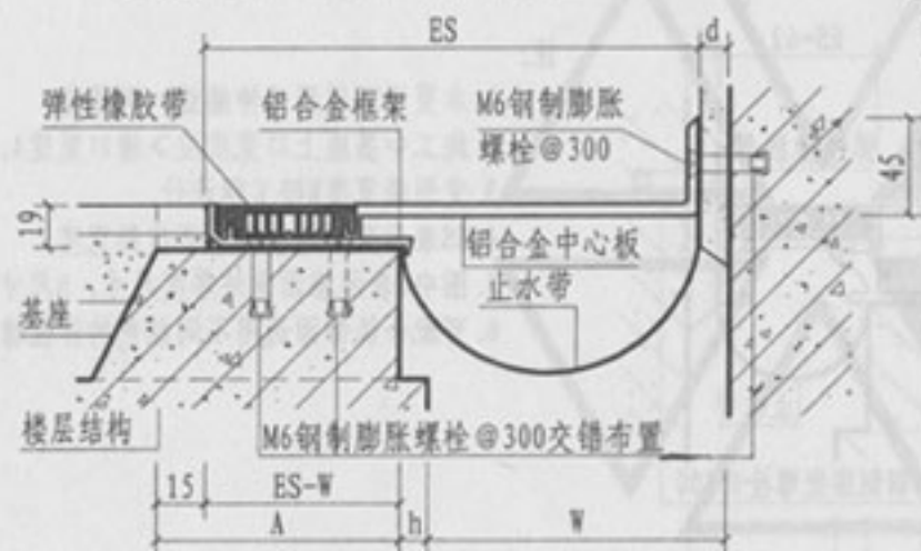
② b 楼、地面与墙面（嵌平式DJR）
