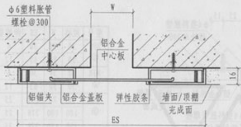
① 内墙/顶棚 (卡锁式 NPK)
