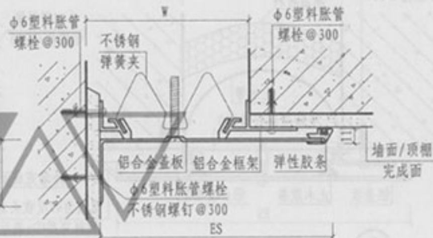
② 内墙/顶棚 (盖板型 NJC)
