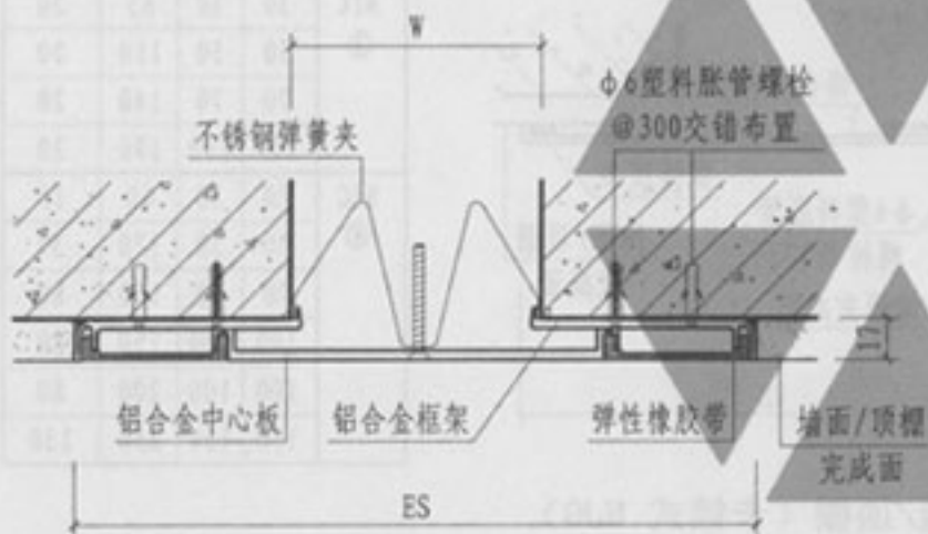
③ 内墙/顶棚（嵌平式 NPRC）
