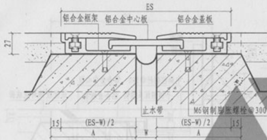
① 楼、地面（承重型DPZL）
