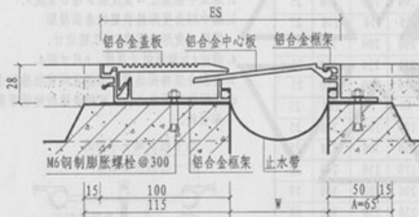
③ 楼、地面（卡锁式DPC）
