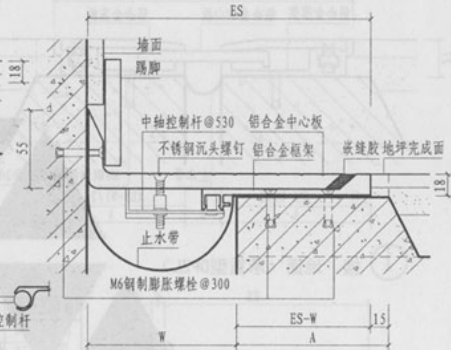
②a 楼、地面与墙面（承重型DJZH）
