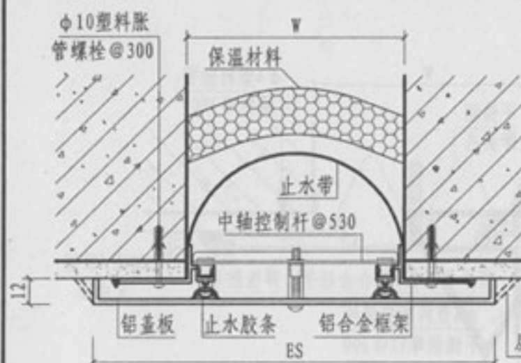
① 外墙 (盖板型 WQPL)
