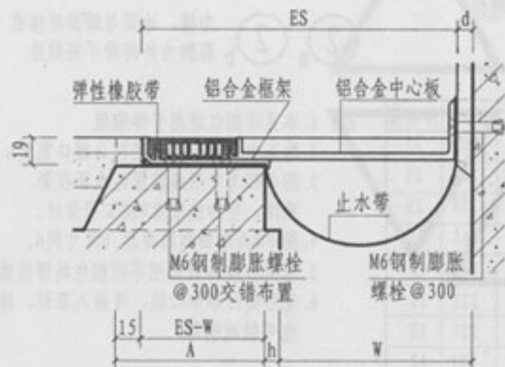
② b 楼、地面与墙面（嵌平式DJRSC）
