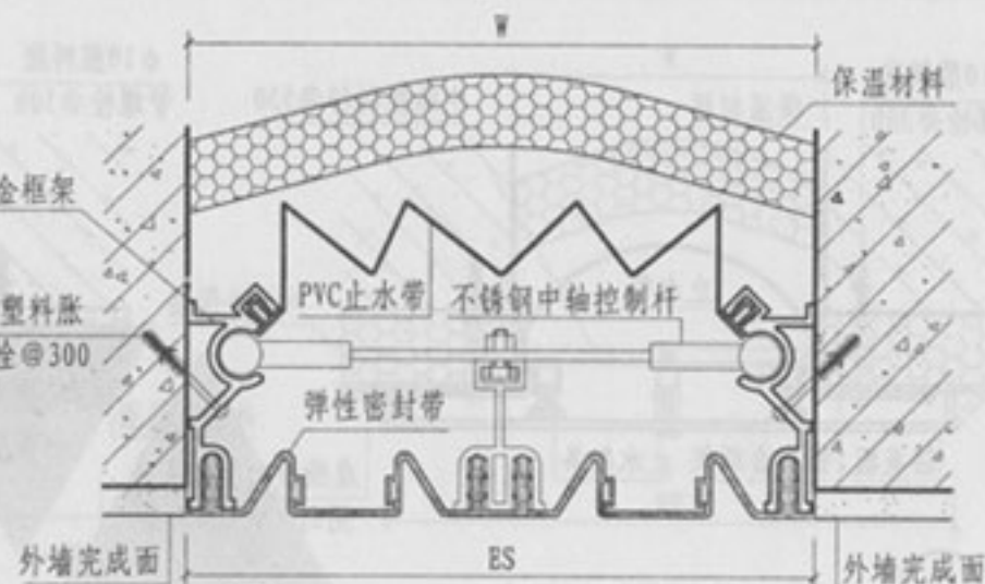
② 外墙（封缝型 WQP） （适合缝宽200-300）
