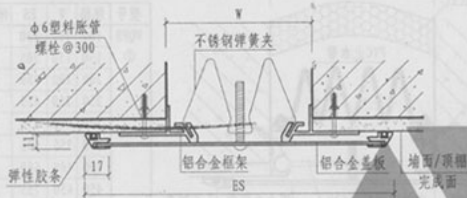
① 内墙/顶棚 (盖板型 NPC)
