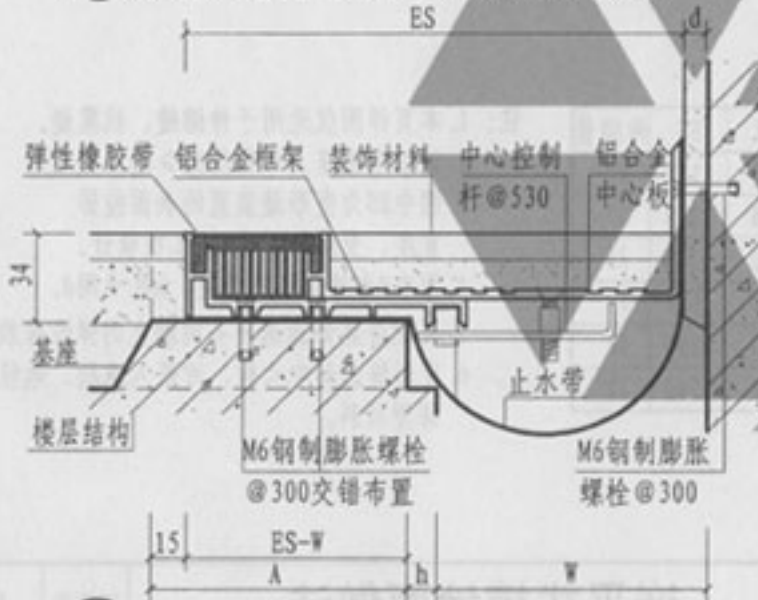
② b 楼、地面与墙面 (嵌平式DJRS)
