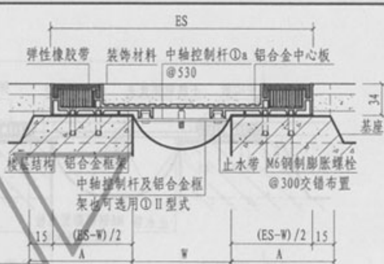
① a 楼、地面 (嵌平式DPRS)
