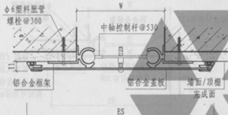
③ 内墙/顶棚 (盖板型 NPH-II)
