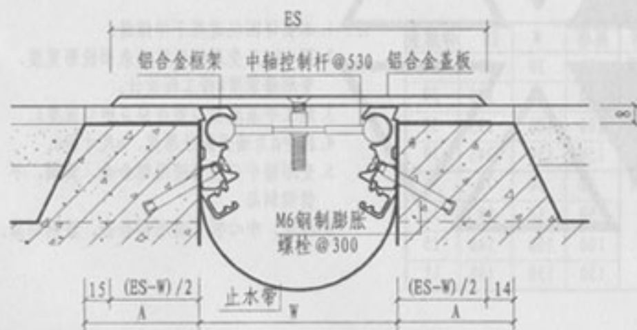
② 楼、地面 (盖板型DPLH)
