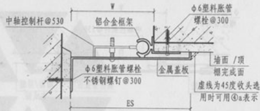
④ 内墙/顶棚 (盖板型 NJL-II)
