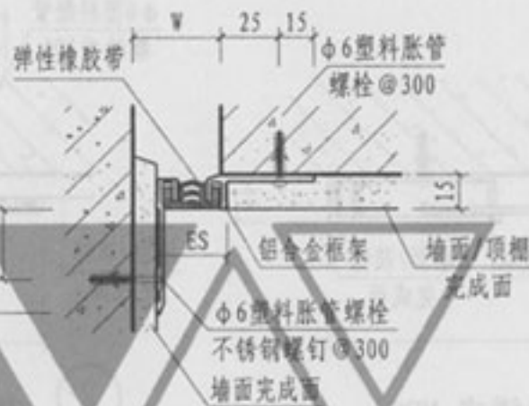
② 内墙/顶棚（嵌平式 NJR）
