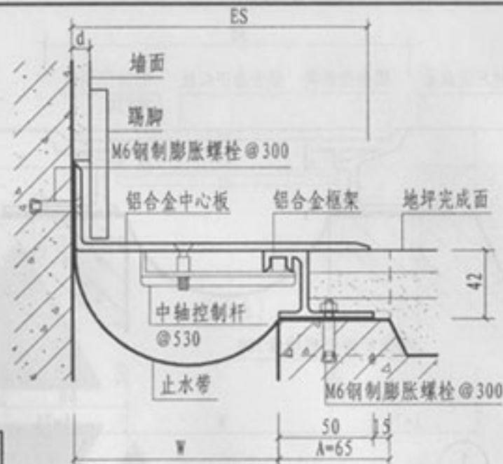
② a 楼、地面与墙面（盖板型DJL）
