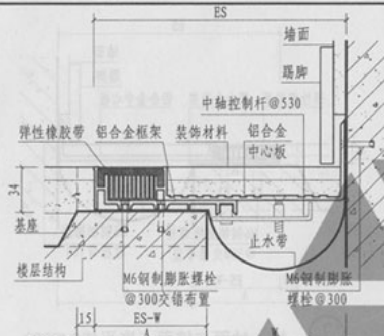
② a 楼、地面与墙面 (嵌平式DJRS)
