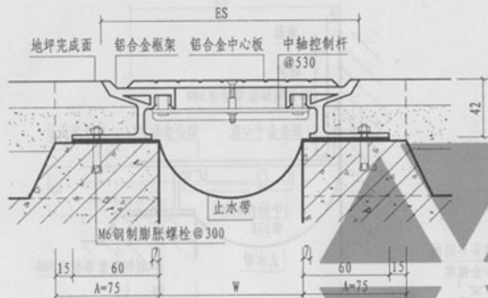
① 楼、地面 (防滑型DPF)
