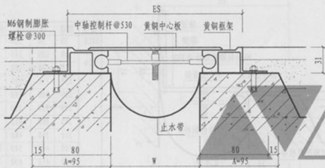
① 楼、地面（盖板型DPPT）
