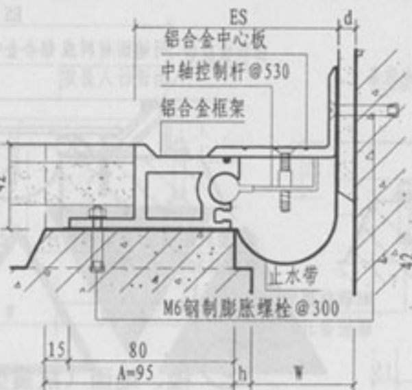
② a 楼、地面与墙面 (承重型DJZG)
