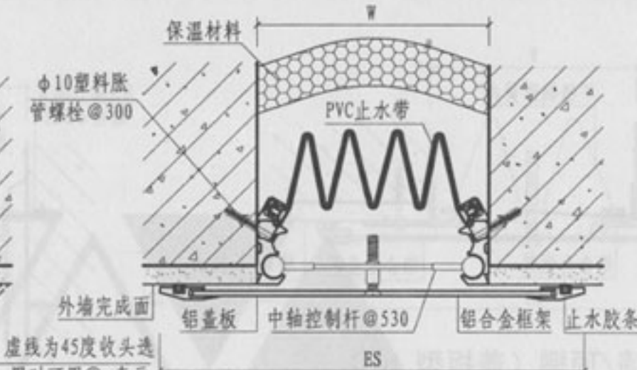
② 外墙 (盖板型 WQPH)
