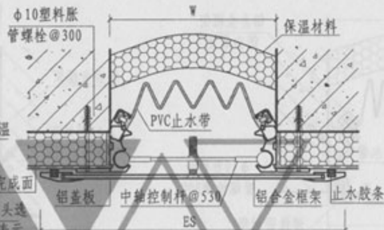
② 外墙 (盖板型 WQPH)
