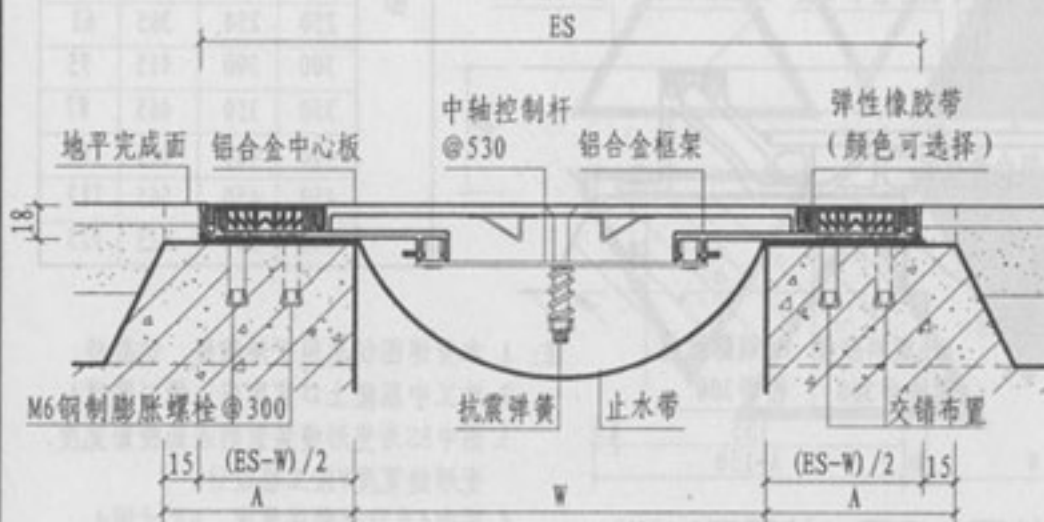
③ 楼、地面 (抗震型DPRM)
