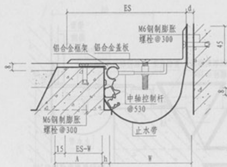
① a 楼、地面与墙面 (盖板型DJLH)
