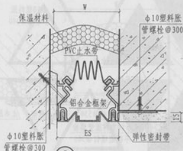
③ 外墙（封缝型 WQJ）
