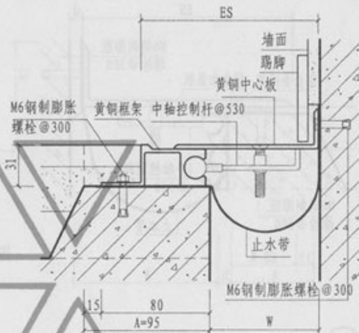
②a 楼、地面与墙面（盖板型DJPT）
